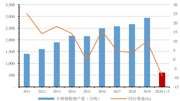
图 3：近年来我国不锈钢粗钢产量及增速情况
