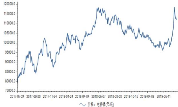
图5：电解镍价格走势情况
