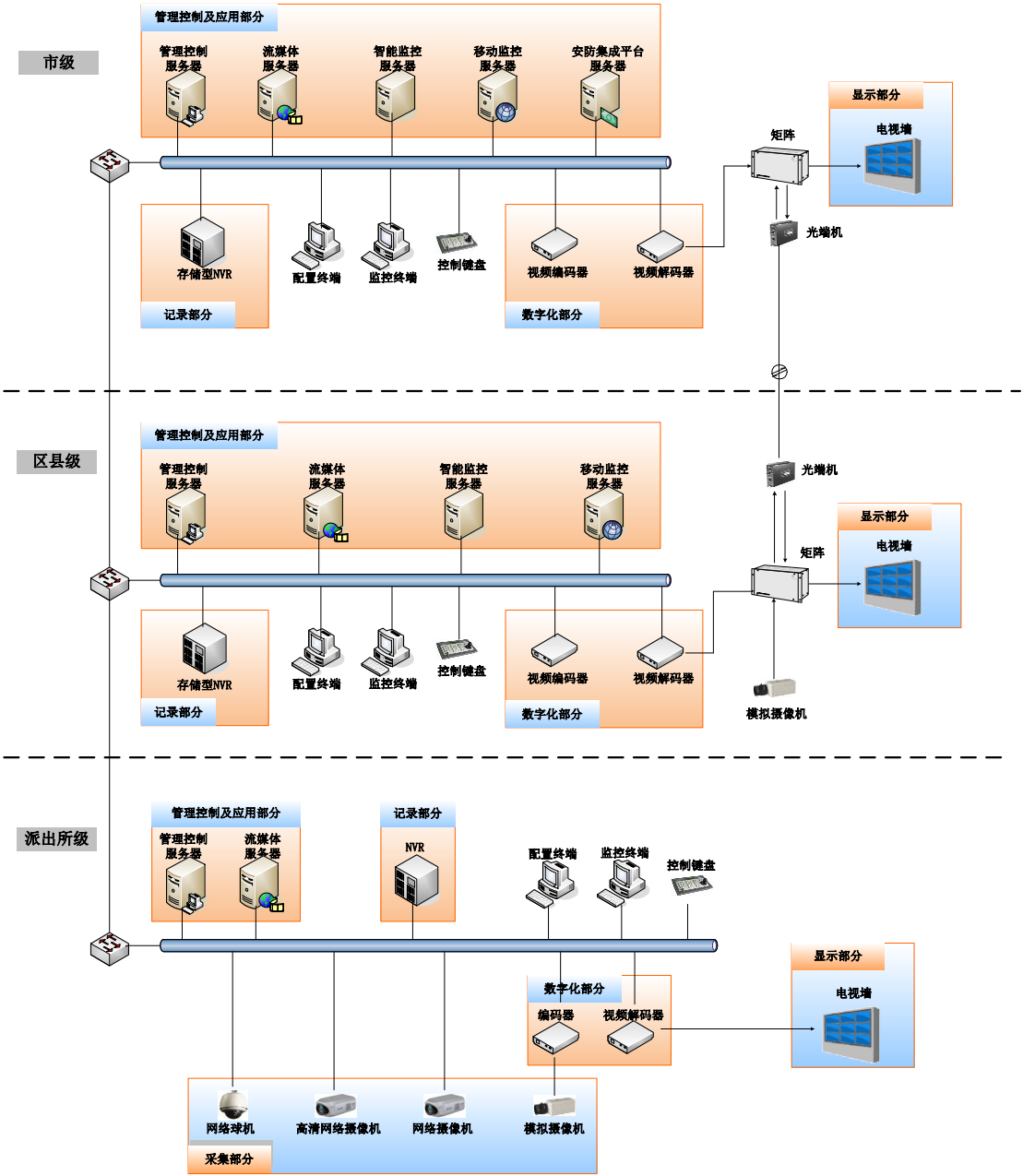
典型城市视频监控系统拓扑图
